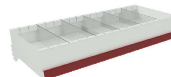
SUPORTE SEPARADOR #20 C/ LATERAL AÇO 92,5x35x10cm - 61551361 130x35x10cm - 61551362 *Bandeja e Divisórias PS não inclusos
