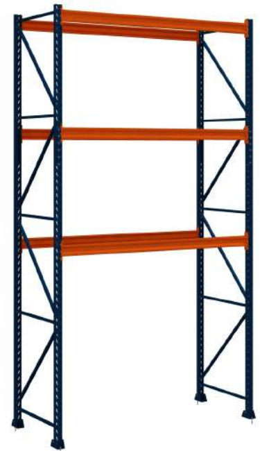
PORTA PALETES 450 x 230 x 100cm C/ 03 NÍVEIS
