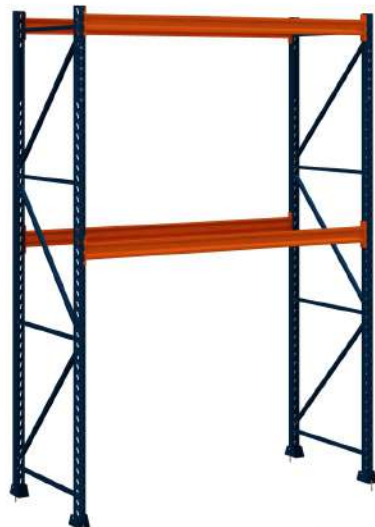
PORTA PALETES 350 x 230 x 100cm C/ 02 NÍVEIS
